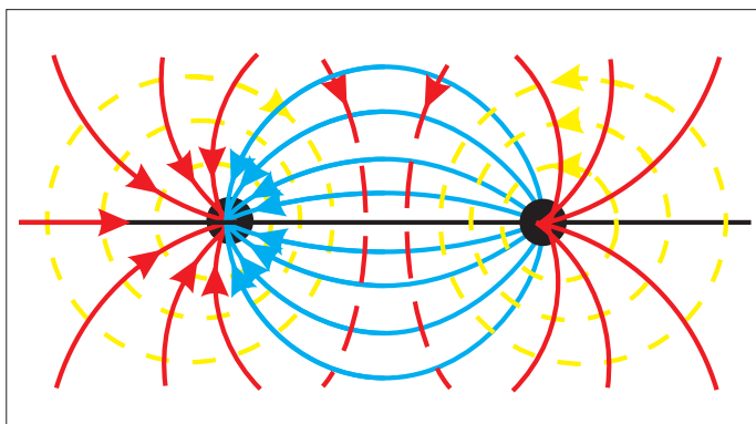
Рис. 1. Принцип действия генераторов поля
